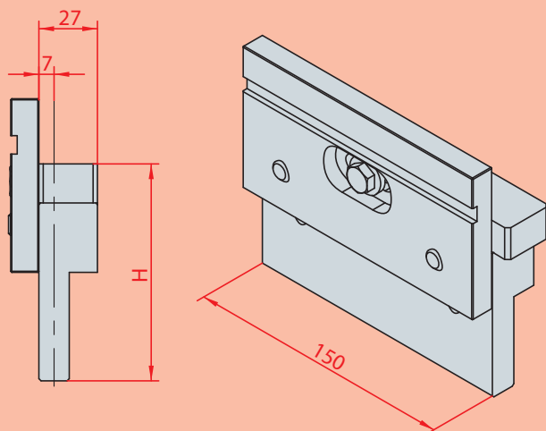
4221 H=100 mm
