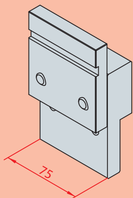
4227 H=150 mm
