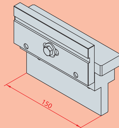
4225 H=120 mm
