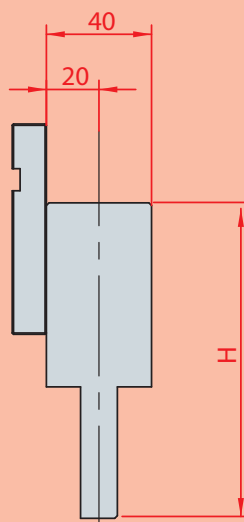
4228 H=120 mm
